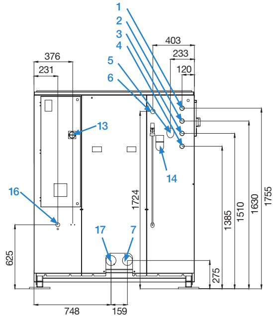
RÜCKANSICHT TWE60
